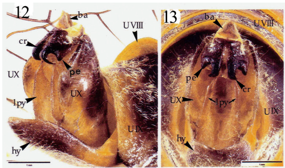
Fig. 12 et 13 : Pomponia matijai n. sp., Holotype mâle, aspect et nomenclature des genitalia externes, vus de profil (12), puis de l'arrière (13). Explication des lettres : b a, bloc anal ; Hyp, hypandrium, ou sternite 8 ; l py, lobes pygophoriens ; U VIII, urite 8 ; U IX, urite 9, ou phallicophore (uncus) ; UX, urite 10, ou pygophore. [Paris, LF Photos].
