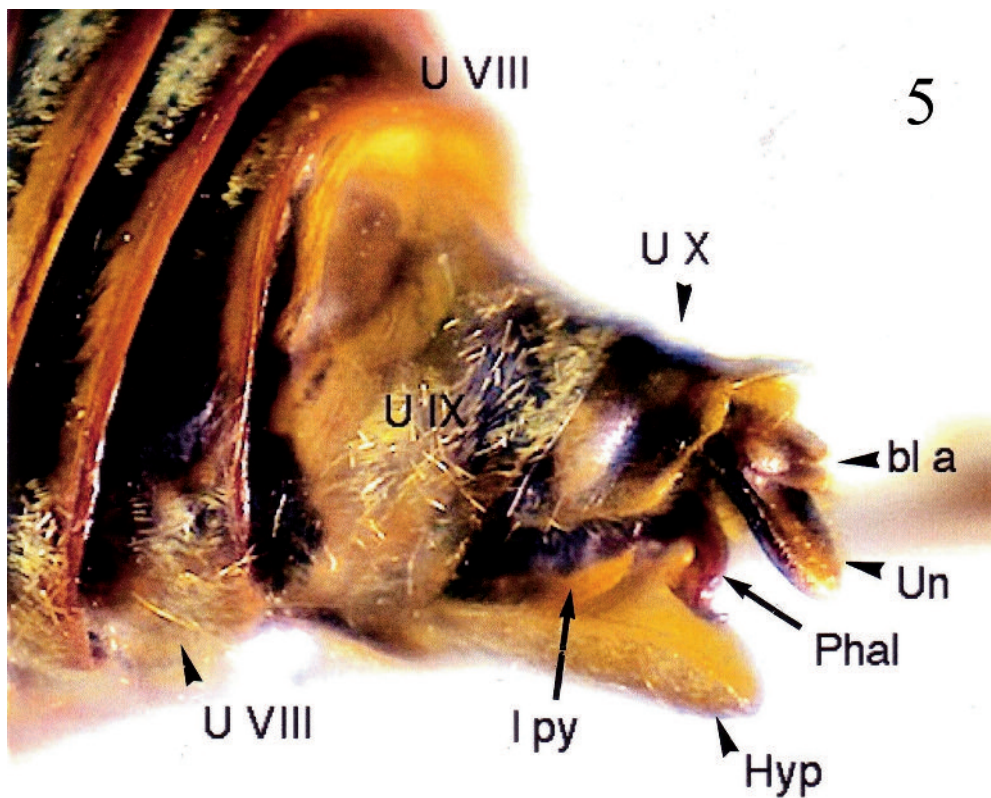
Fig. 5 : Malagasias gogalai n. sp. Paratype ♂. Vue rapprochée de l'apex génital légèrement ouvert : bl a, bloc anal ; Hyp, hypandrium ; l py, lobe pygophorien ; PC, processus caudal ; Phal, phallus ; Un, phallicophore (uncus) ; U VIII, urite 8 ; U IX, urite 9 ; U X, urite 10, ou pygophore (Microphotographie MB).
