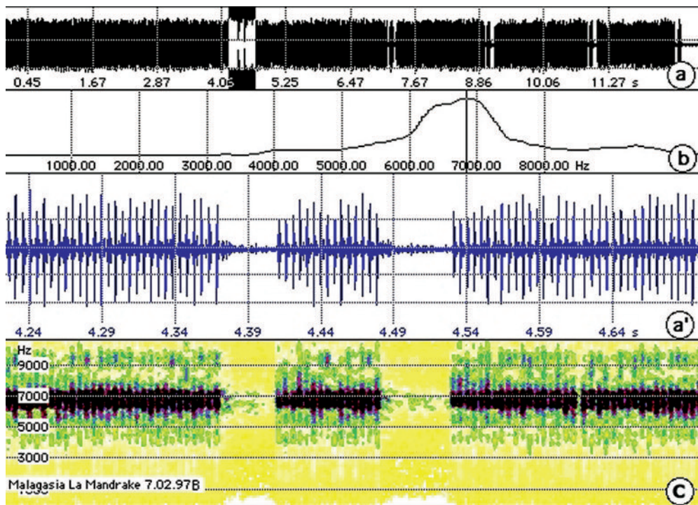
Fig. 7 : Malagasias gogalai n. sp. MB CIA, Carte d'identité acoustique indicative, ainsi commentée :
