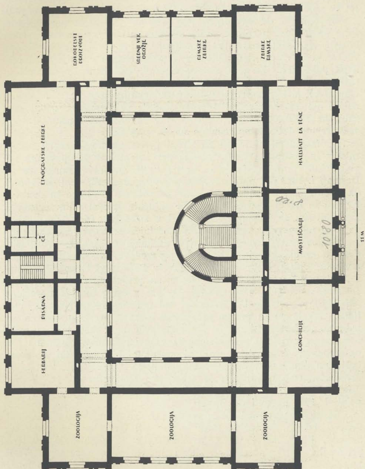
Muzejska zgradba: Tloris I. nadstropja
