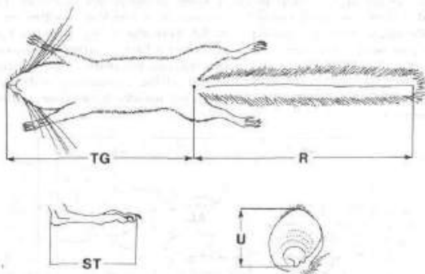
Slika 3: Način merjenja sesalca. TG – dolžina trupa z glavo, R – dolžina repa, ST – dolžina stopala, U – dolžina ušja.
