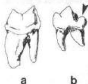
Slika 145: Prvi spodnji meljak pri (a) mačkah ( Felidae ) in (b) psih ( Canidae ). Puščica kaže zadnji sploščen del zoba, ki je še namenjen mletju.
