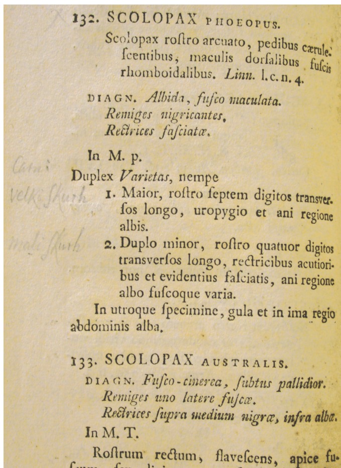
Slika 3. Zoisovi pripisi.
